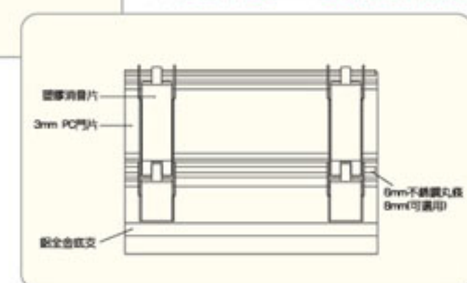
◀◀◀ 鋁合金 PC 透明門片結構圖
