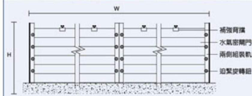
鋁合金防水閘門示意圖
