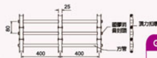
GS-80 不銹鋼方管花格門片結構圖
