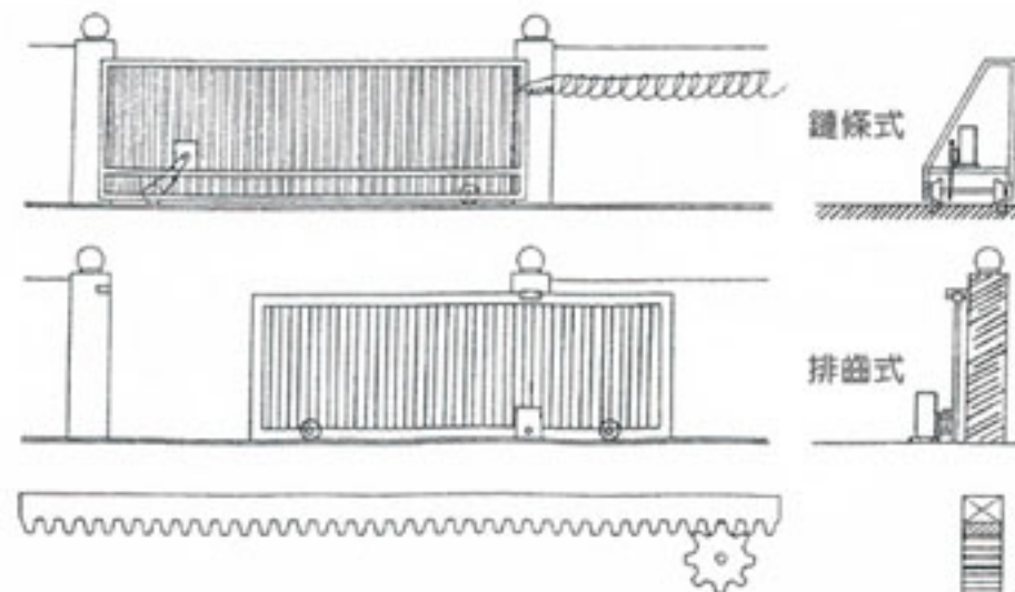
車庫門 尺寸示意圖 >>>
