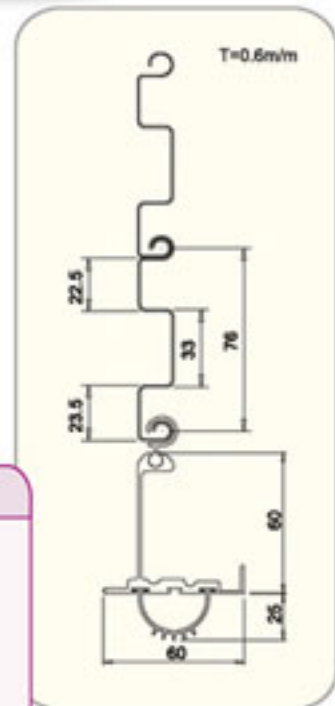
不銹鋼捲門片結構圖
