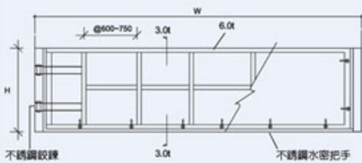
不銹鋼防水閘門示意圖
